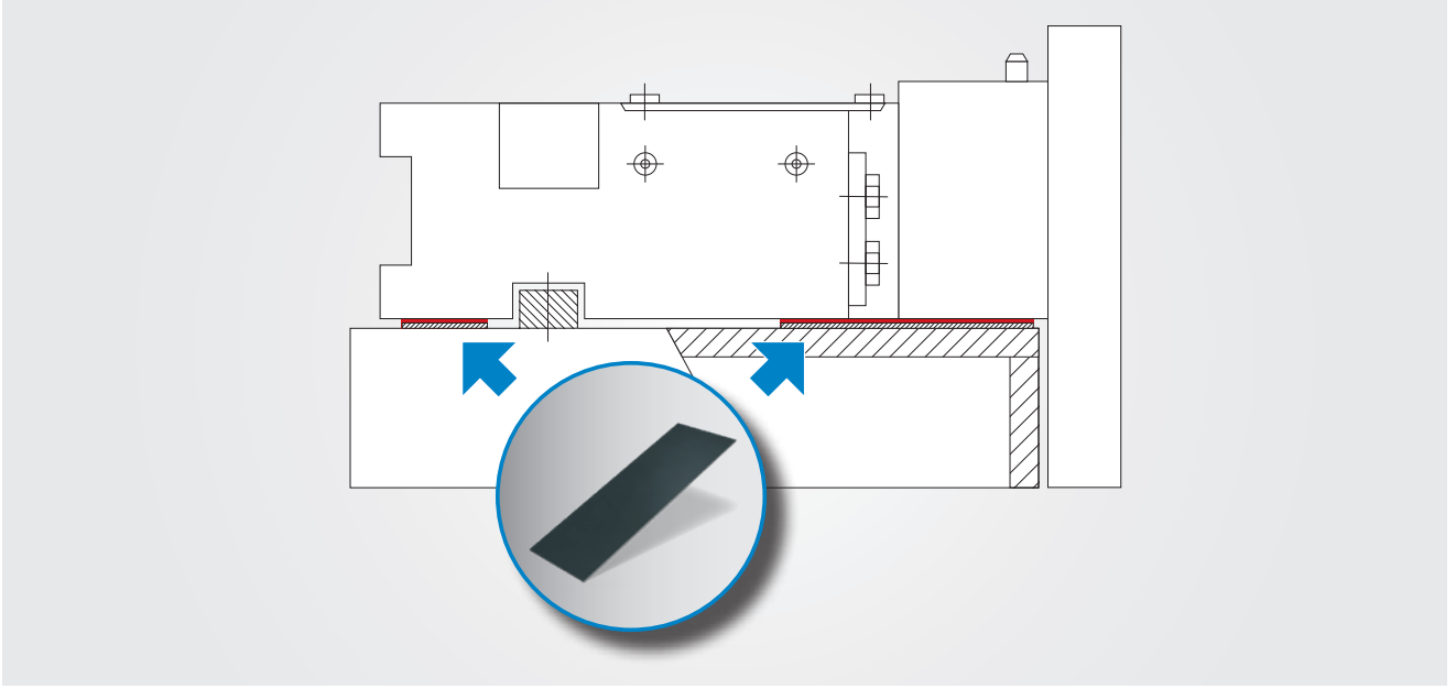
Permaglide® Yapı türü PAS ... P180 kaymalı şeritlerin olduğu bir kızak kılavuzundaki yataklamlar
